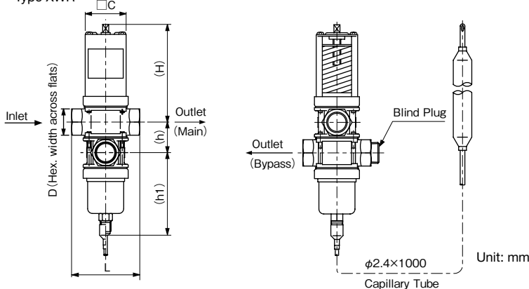
Type XWR
