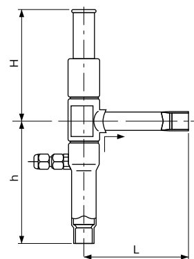
Type EPR-D
