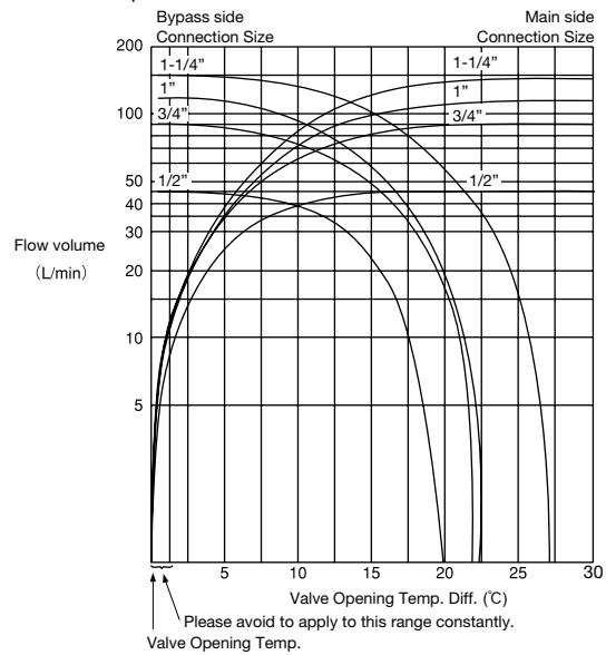
Type XWR
