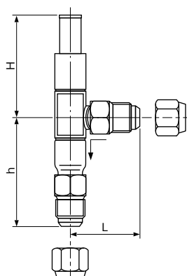
Type SPR-B
