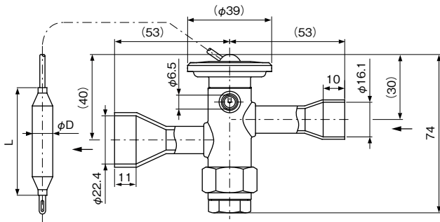
Type SCX-57D
