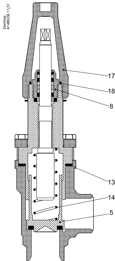
Fig. 1, SCH 15-40
