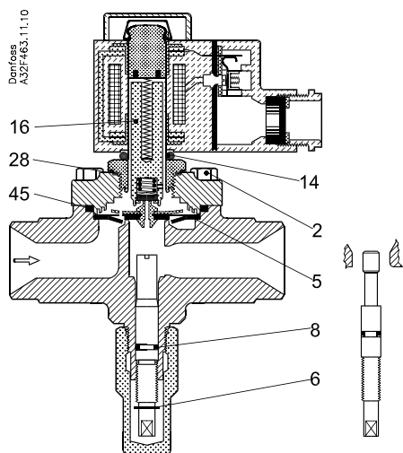
Fig. 1, EVRS 10, 15 and 20
