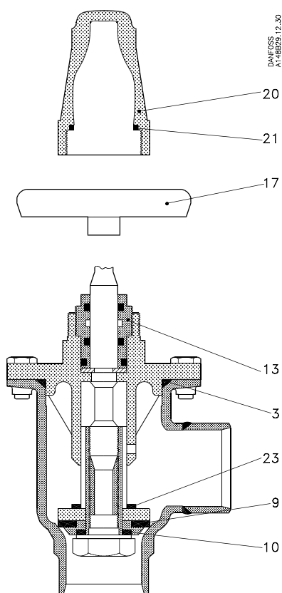
Fig. 1, SCV 25-200
