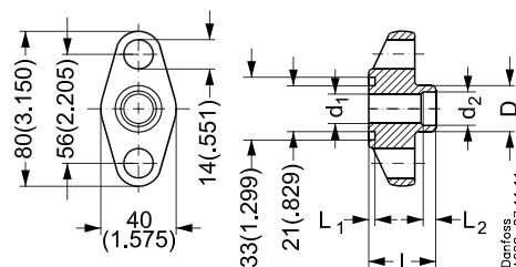
Groove flange
