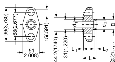
Groove flange
