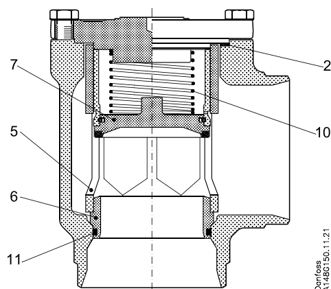
Fig. 1, CHV 50 - 125
