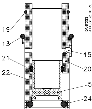
Fig. 2, Guide piece
