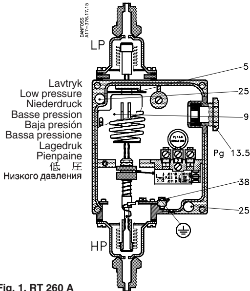
Fig. 1. RT 260 A
