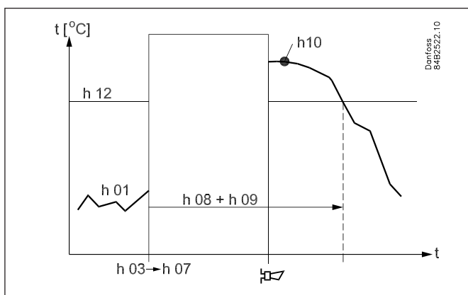
Przekroczenie limitu w przypadku zaniku napięcia zasilającego przez czas nieprzekraczający czasu podtrzymania zegara wewnętrznego sterownika.
