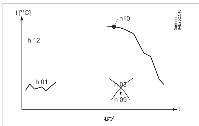
Przekroczenie limitu w przypadku zaniku napięcia zasilającego przez czas przekraczający czas podtrzymania zegara wewnętrznego sterownika. Sterownik nie może tym samym zapamiętać parametrów związanych z czasem trwania przekroczenia.
