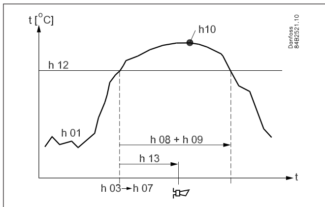
Przekroczenie limitu w czasie normalnej pracy
