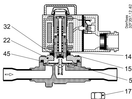
Fig. 2, EVRC 20 (NO)
