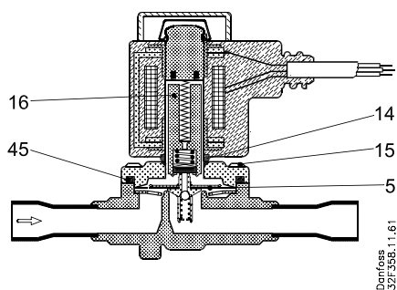
Fig. 1, EVRC 20 (NC)
