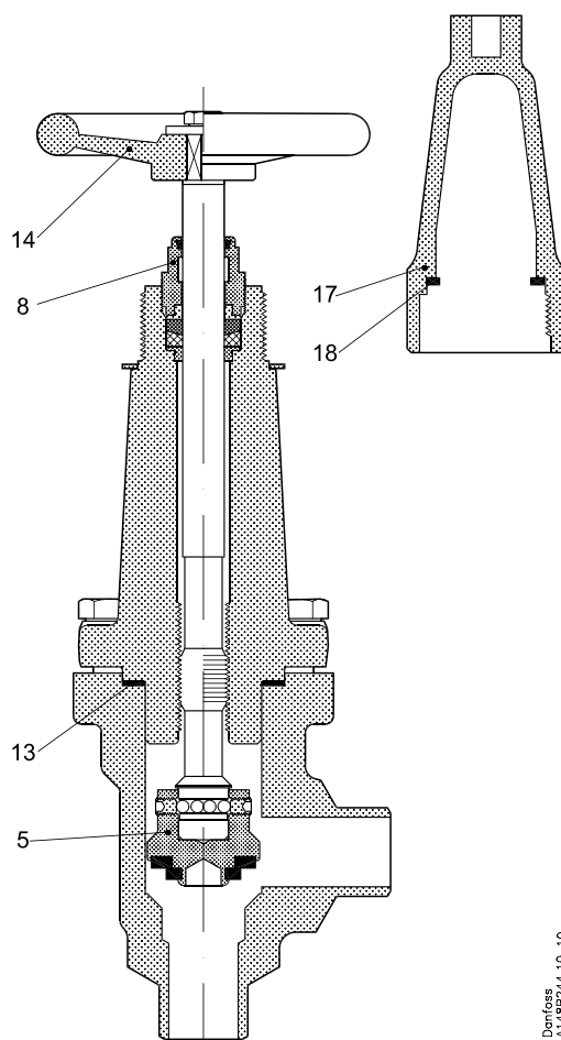
Fig. 1, SVA-HS 15-40
