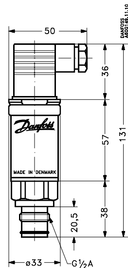
Stikudførelse DIN 43650 Pg 9
